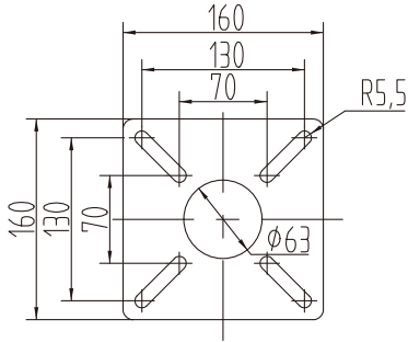
24L/30L 电眼料斗（默认大底座） 24L/30L Sensor hopper (large base)
